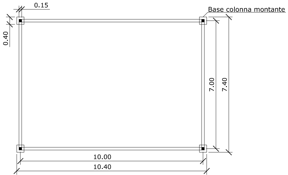
- PIANTA
